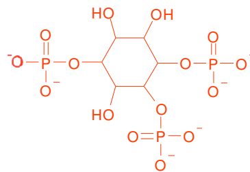
Inositol 1,4,5-trisfosfato (InsP 3 ) Estimula la liberación de Calcio desde el retículo endoplásmico
